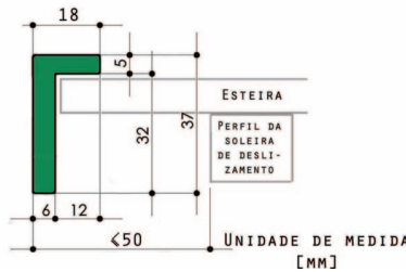
PERFIL PARA ESTEIRAS CURVAS SEM LINGUETA PL 32-18-6
