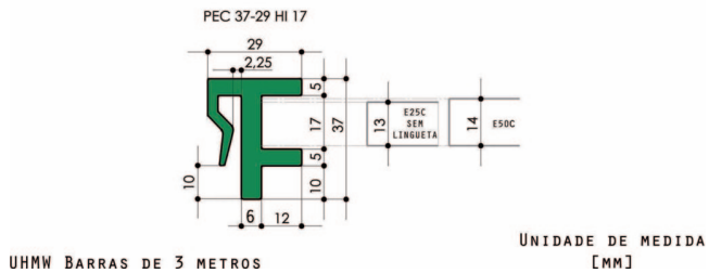
PERFIL CLIP PARA ENCAIXE EM CHAPA COM ESPESSURA DE 2,5MM ATÉ 4,76MM
