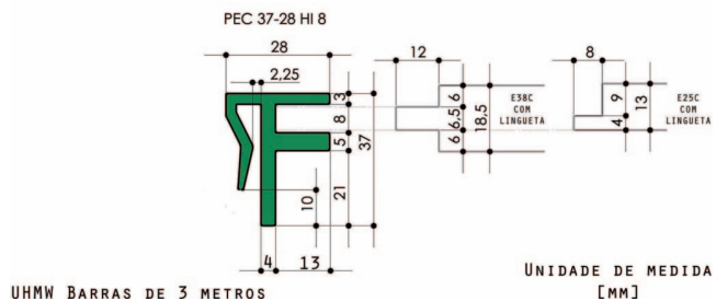
PERFIL CLIP PARA ENCAIXE EM CHAPA COM ESPESSURA DE 2,5MM ATÉ 4,76MM
