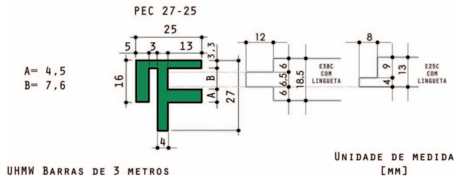
PERFIL PARA ENCAIXE EM CHAPAS DE ESPESSURA DE 3MM
