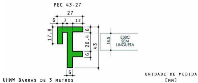
PERFIL PARA ENCAIXE EM CHAPAS DE ESPESSURA 3MM (1/8")
